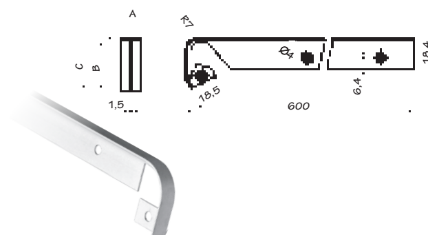
Spojnice radne ploče / šteljući nastavak
