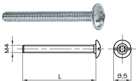
Šraf za ručice / M4
