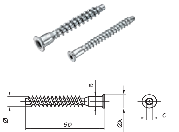
Iver vijak (confirmat)
