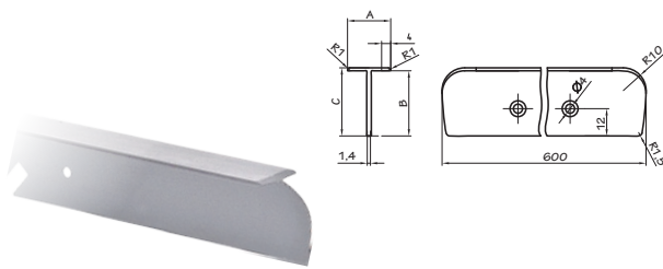
Spojnice radne ploče / nastavak
