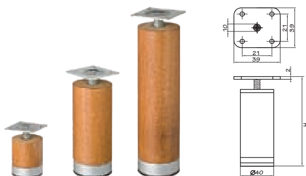
Nogica RONDO / trešnja
