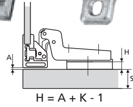
Klap šarka za alu-profil / M Slide-On / FGV
