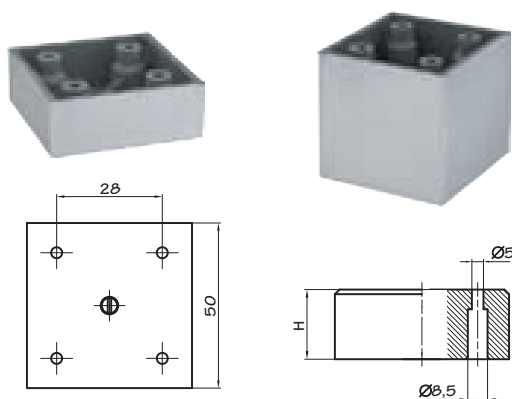
Fiksna stopica / Cuba
