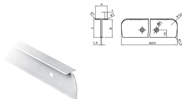
Spojnice radne ploče / nastavak
