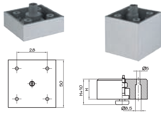
Fiksna stopica / Cuba
