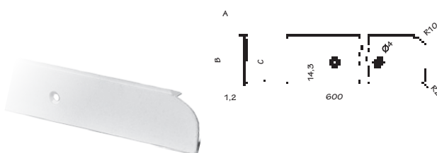
Spojnice radne ploče / završetak / 3cm
