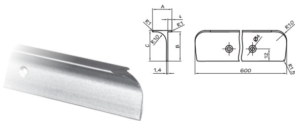
Spojnice radne ploče / ugao
