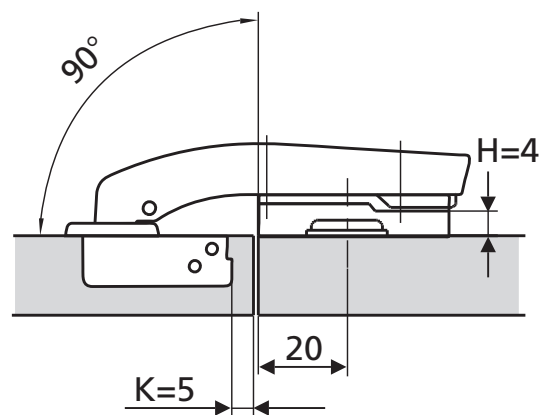
Klap šarka ugaona / 90° / FGV
