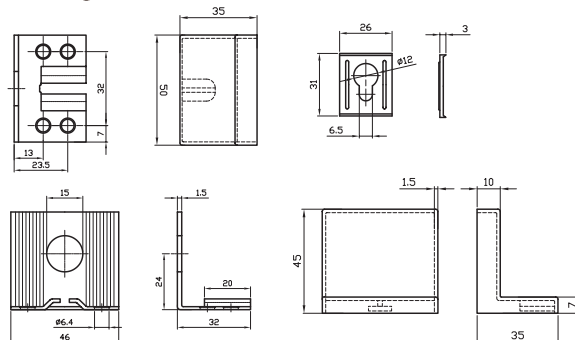
Nosач kuhinjskog elementa / šraf sistem
