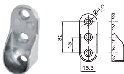
Nosač elipsaste oklagije
