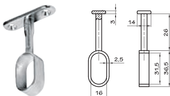
Srednji nosač elipsaste oklagije
