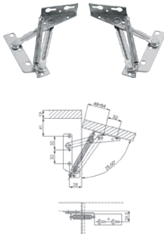
Šarka sa oprugom
