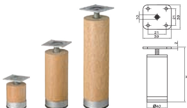
Nogica RONDO / bukva
