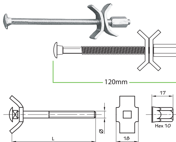
Spojni okov za radne ploče
