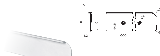
Spojnice radne ploče / završetak / 4cm
