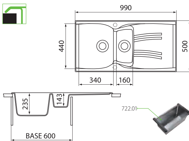
Granitna sudopera NK 9910
