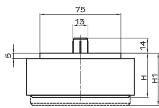
Nogica POLIPLAST / 704 R
