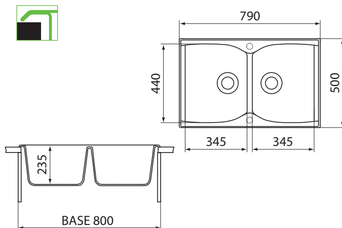
Granitna sudopera NK 7920
