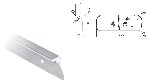
Spojnice radne ploče / ugao
